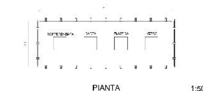
DIMENSIONE CASSONETTI 1.700 LITRI 1:50
