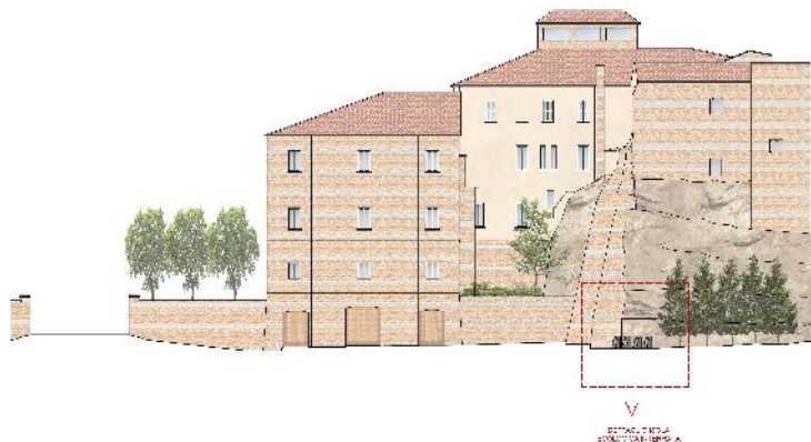
PROSPETTO LATO STRADA PROVINCIALE 17 - INTERVENTI DA REALIZZARE
